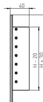
VISTA LATERALE SCALA 1:2
