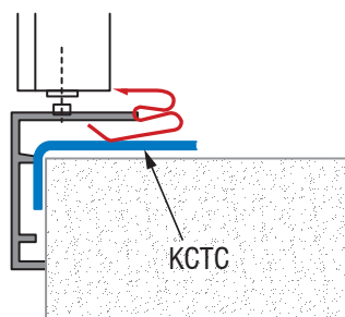
Standard FISSAGGIO CON CLIPS
