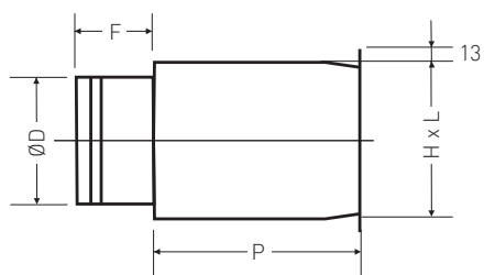
PBOS-PB0I Plenum con attacco posteriore
