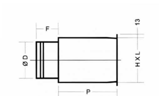
PBOS-PBOI PLENUM CON COLLARINO ORIZZONTALE
