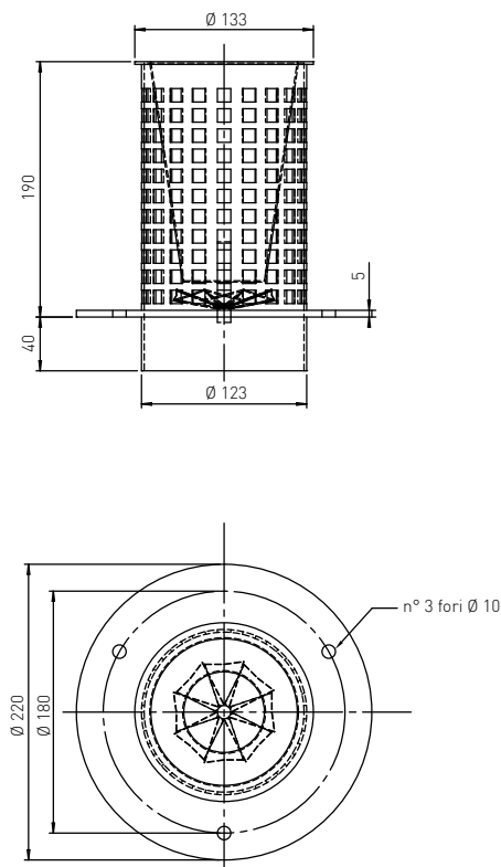
DIFFUSORE STANDARD
