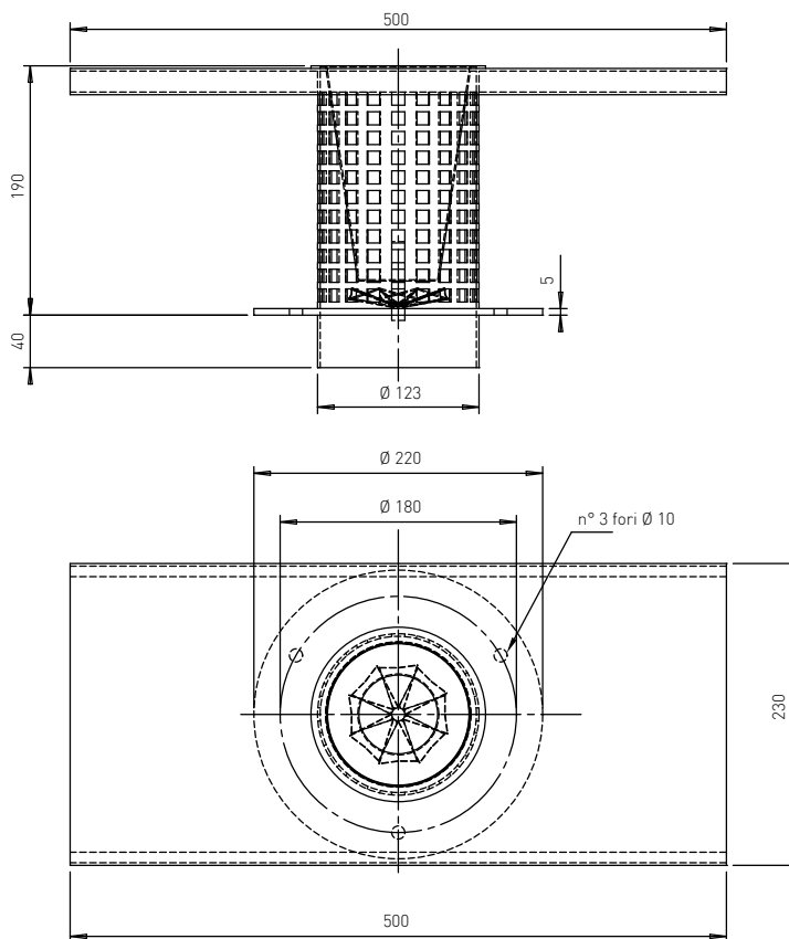
DIFFUSORE CON PIASTRA DI SUPPORTO
