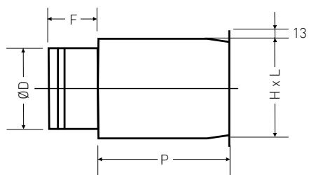
PB0S-PB0I Plenum con attacco posteriore
